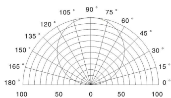
Distribución luz
