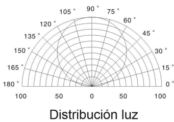
Distribución lumínica
